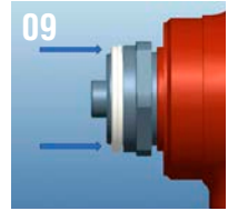
9.- 手动完成将唇形密封圈插入槽口喷嘴
